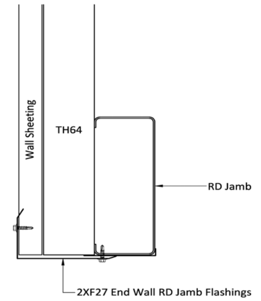
End Wall RD Jamb Flashing 2XF27/18
